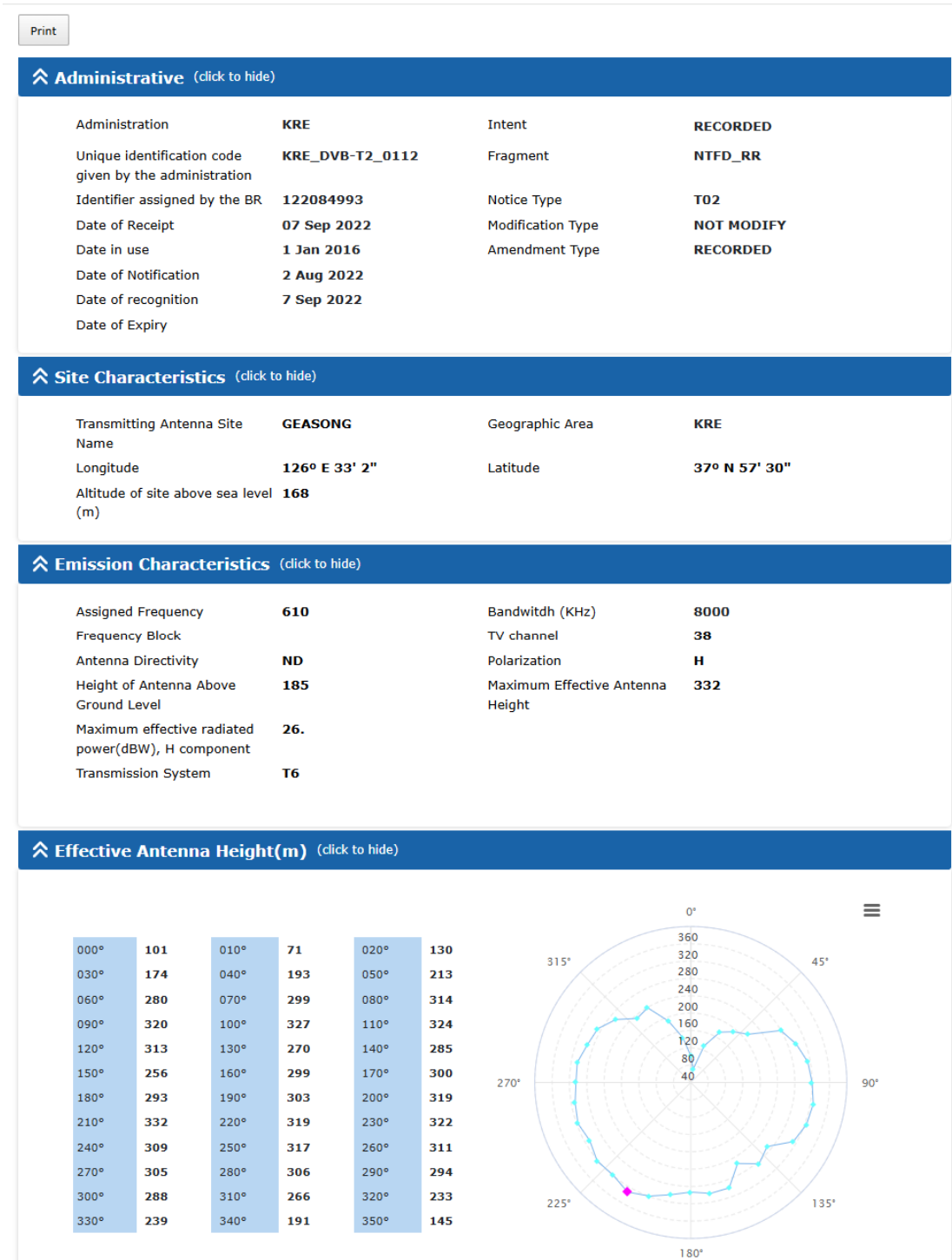
그림 3. ITU eMIFR(broadcasting)에 등록된 개성중계소 DVB-T2 디지털 송신 제원 상세
