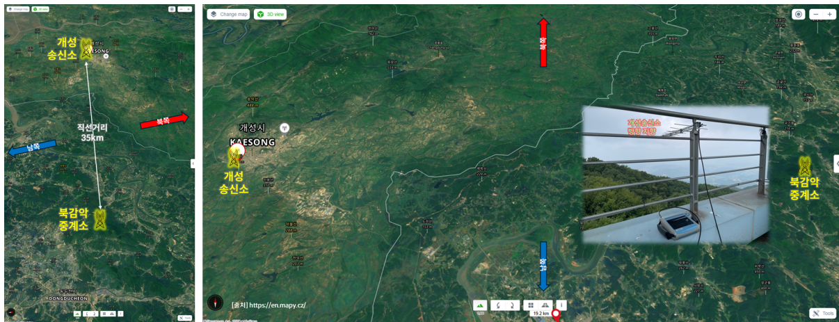
그림 5. 개성중계소 송신-북감악중계소 수신 구간 직접 수신 환경 분석. 직선거리 35km 가량 됨 Fig. 5. Analysis of Direct Reception Environment between Gaeseong Transmitter and Bukgamak Station Receiver – Approximately 35 km Line-of-Sight Distance
