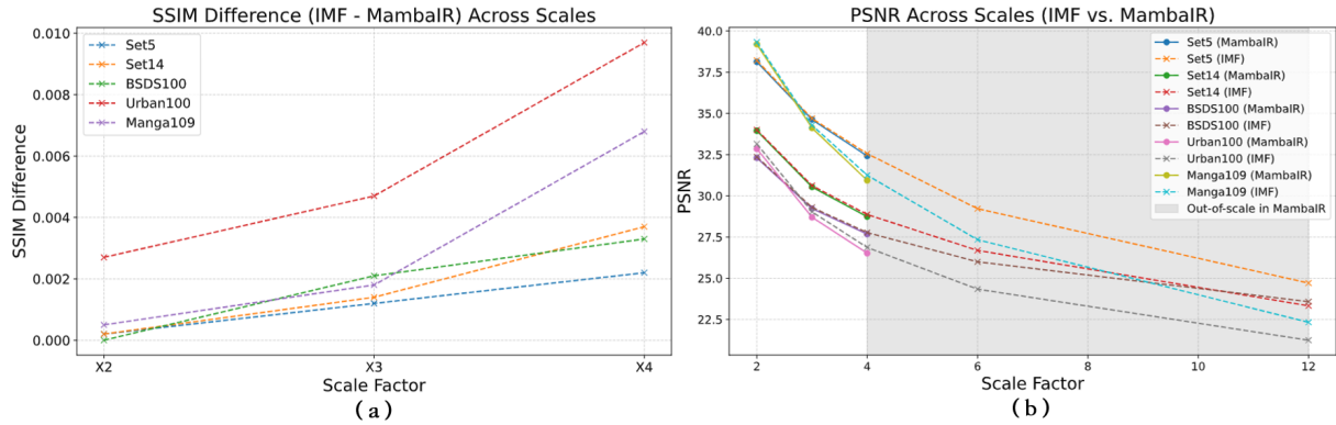
그림 2. (a) 스케일 증가에 따른 SSIM 차이(IMF - MambaIR) (b) 다양한 배율에서의 PSNR 비교(IMF vs MambaIR) Fig. 2. (a) SSIM difference(IMF - MambaIR) across scales (b) PSNR comparison across multiple scales(IMF vs MambaIR)
