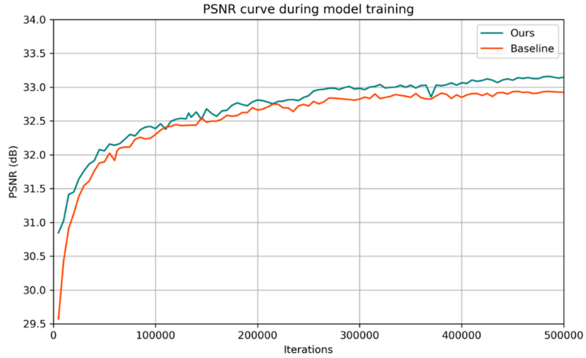
그림 4. 2배율 학습 과정에서의 검증 PSNR 변화 추이 Fig. 4. Validation PSNR Trend during ×2 Scale Training
