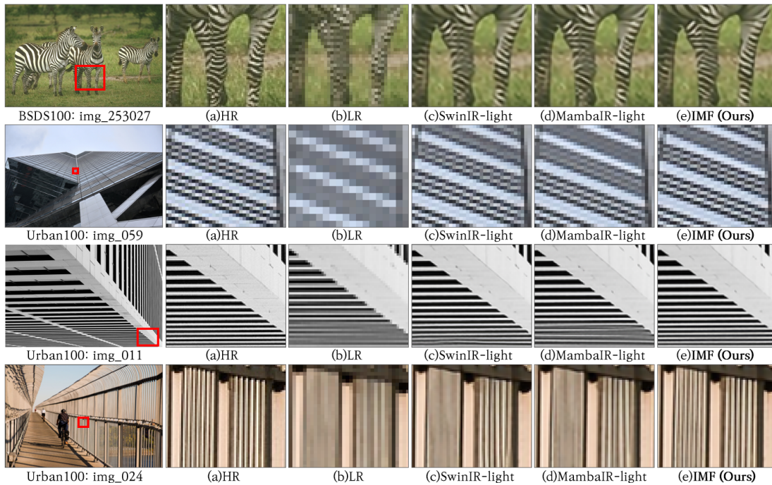
그림 3. 2배율 초해상도 복원 결과의 정성적 비교 (a) HR (b) LR (c) SwinIR-light (d) MambaIR-light (e) IMF(Ours) Fig. 3. Qualitative comparison for x2 super-resolution (a) HR (b) LR (c) SwinIR-light (d) MambaIR-light (e) IMF(Ours)
