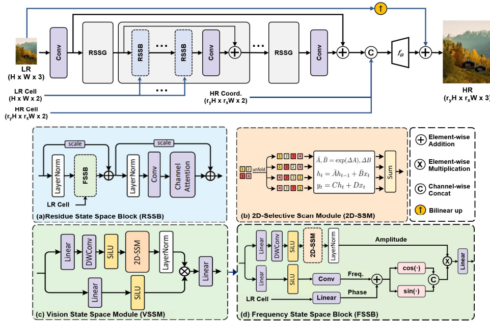
그림 1. IMF 구조 개요 Fig. 1. Overview of the IMF architecture
